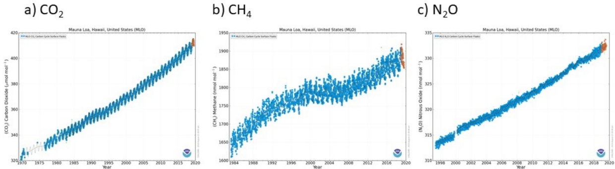
Figure 2. Évolution des concentrations des principaux gaz à effet de serre mesurés à l'Observatoire de Mauna Loa Hawaï (NOAA 2019).
